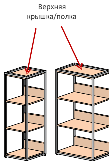
Стеллажи 3 уровня
